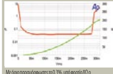
Με άριο παραμόρφωσης το 0,3%, υπό φορτίο 8Ω ο ενισχυτής απέδωσε 2x127 Wrms, ενώ στα 4Ω η τιμή αυτή διαμορφώθηκε στα 2x180 Wrms. Παλλά και καλά Watt και με χαμηλές παραμορφώσεις.
